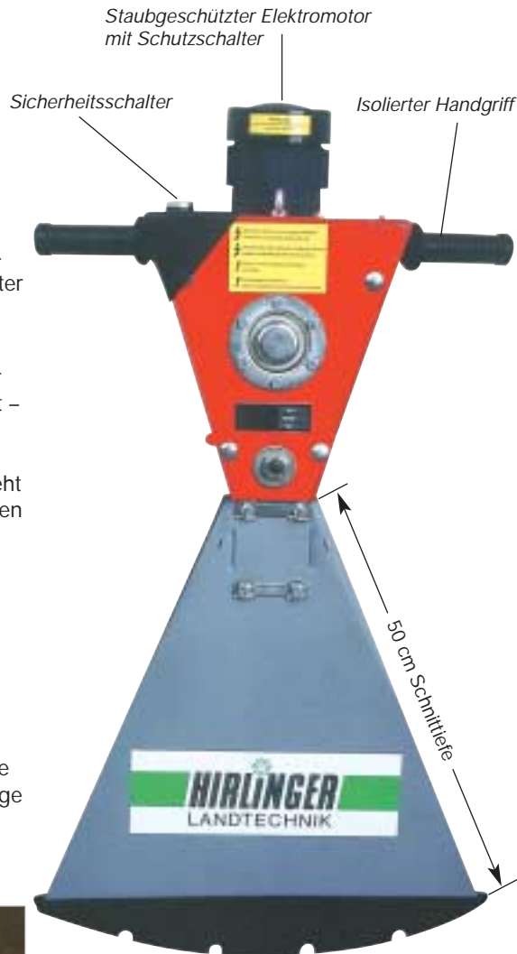
Verschleißarme Sägeklingen, die sich wie bei einer Heckenschere freischwingend gegeneinander bewegen und sich mit hoher Geschwindigkeit ins Futter hineinfressen (Abbildung mit Unfallschutz).
